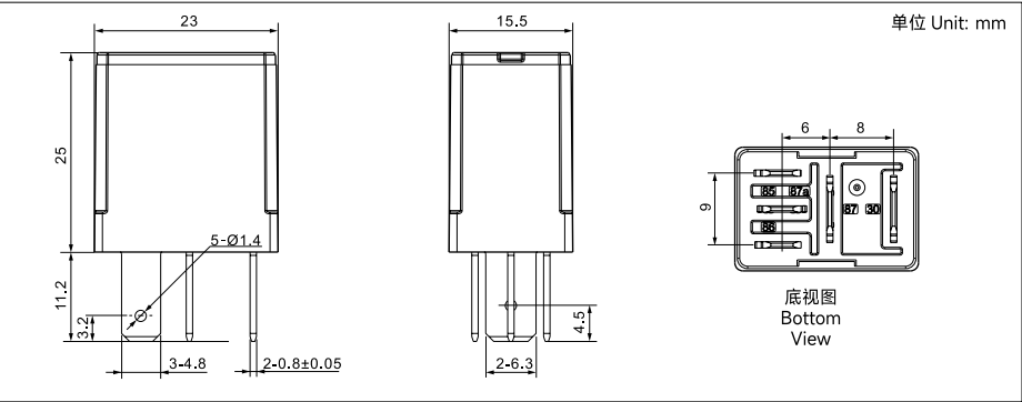
外形尺寸 / 安装孔尺寸 (底视图) OUTLINE DIMENSIONS/PCB LAYOUT (BOTTOM VIEW)
